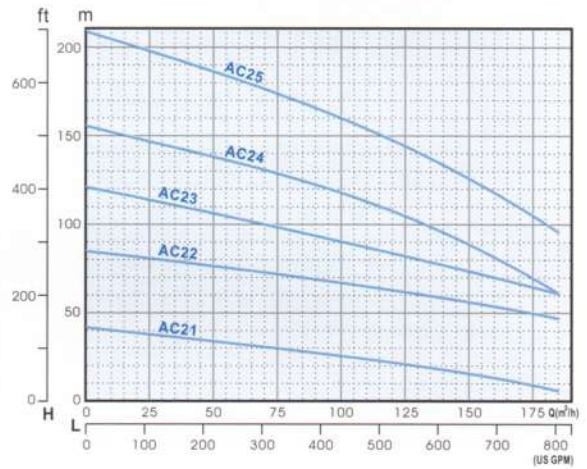
性能曲線表
