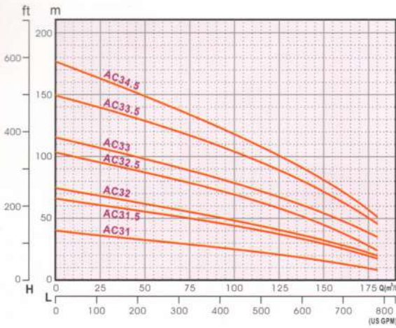
性能曲線表
