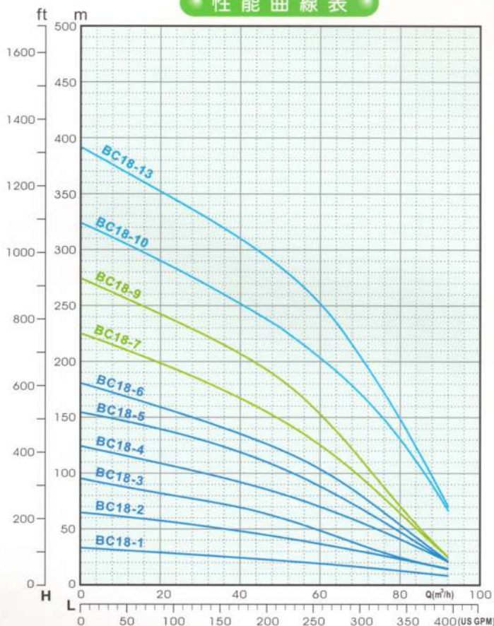
性能曲線表
